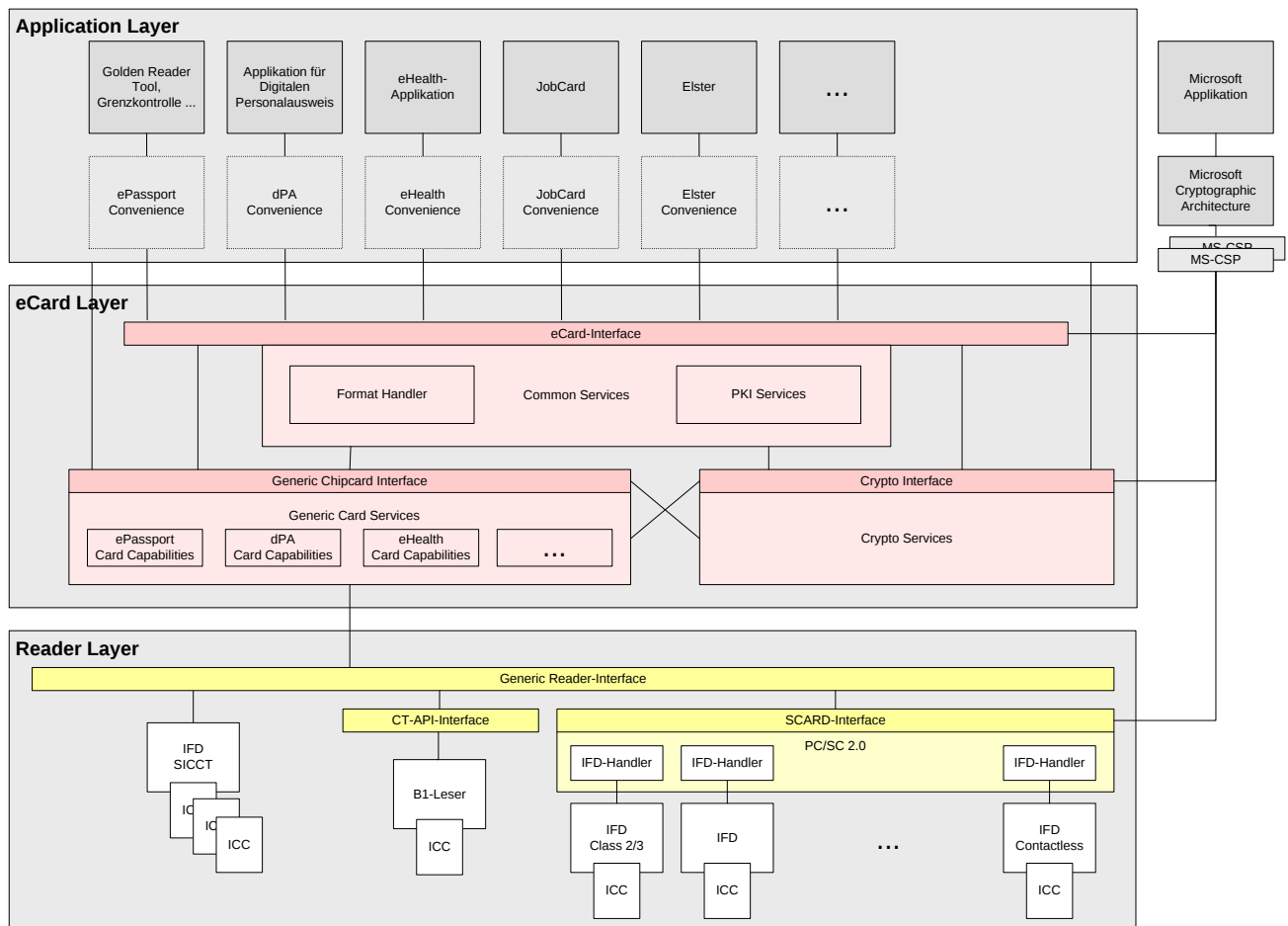
Abbildung 10: eCard-Framework
