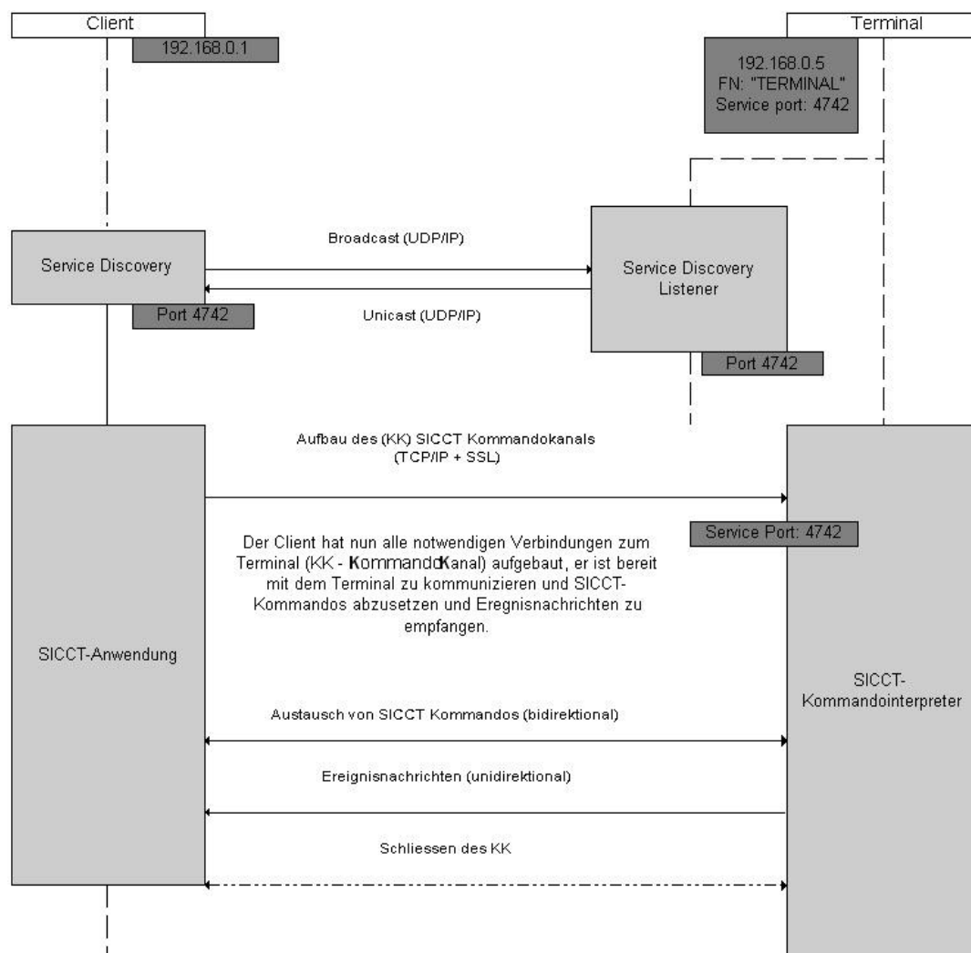
Abbildung 9 SICCT Netzwerkverbindungen
