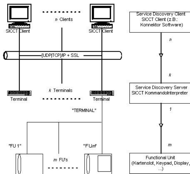
Abbildung 8 SICCT Netzwerkmodell
