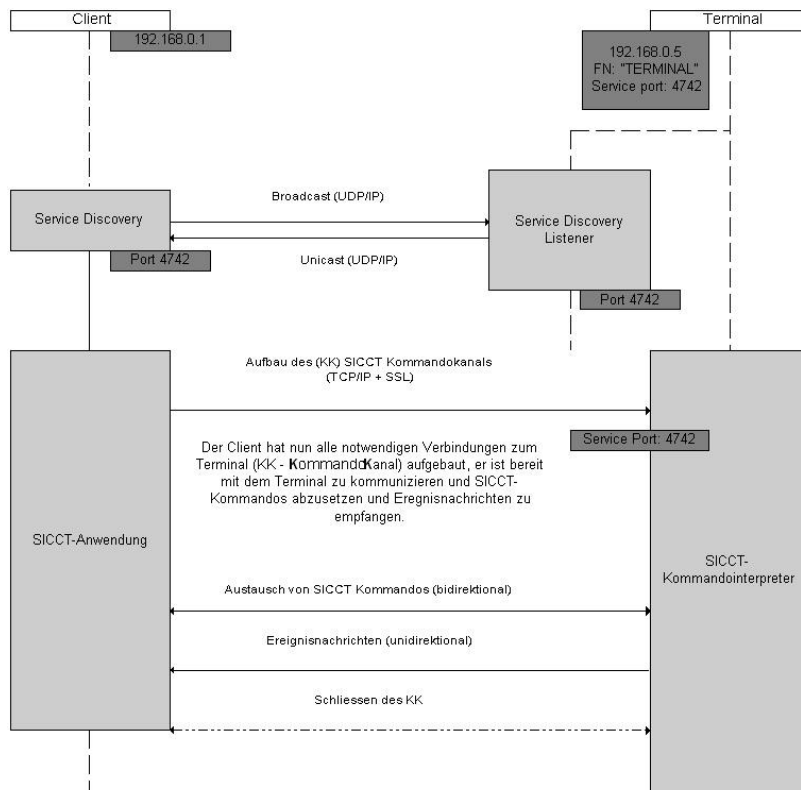
Abbildung 9 SICCT Netzwerkverbindungen
