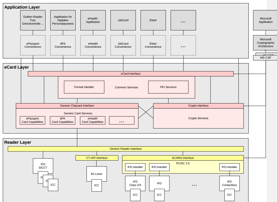
Abbildung 10: eCard-Framework
