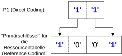
Abbildung 3: Beispielabbildung für Direct Coding auf Ressourcentabelle
