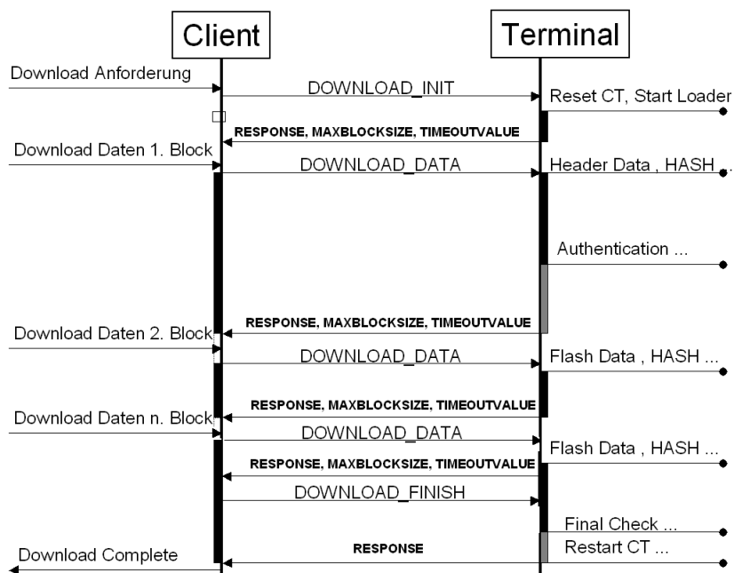
Abbildung 4: Beispielablauf des Firmware-Downloads
