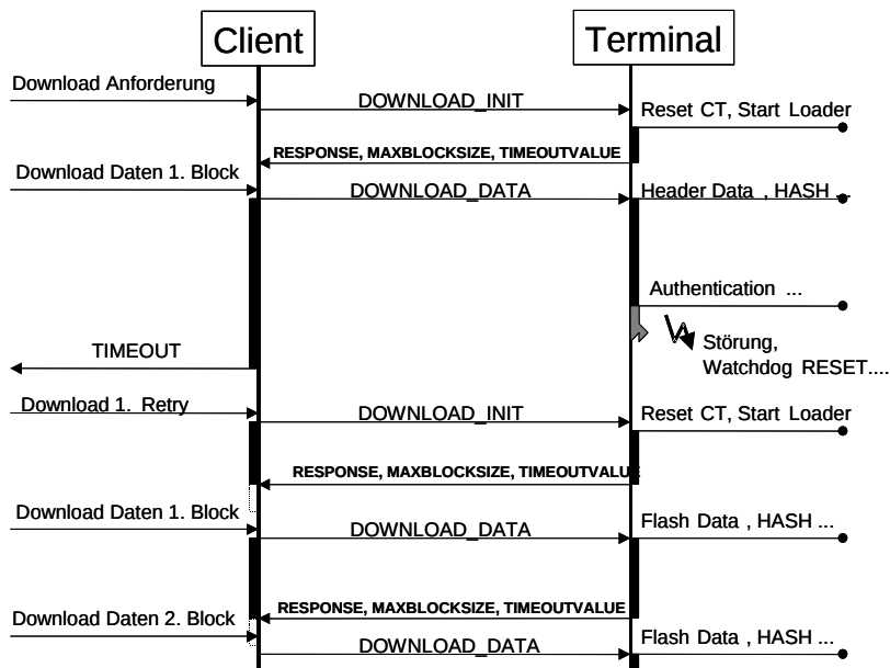
Abbildung 5: Beispielablauf der Fehlerbehandlung beim Firmware-Download
